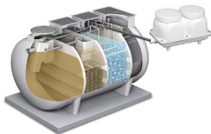
浄化槽(分散型汚水処理) PV型
