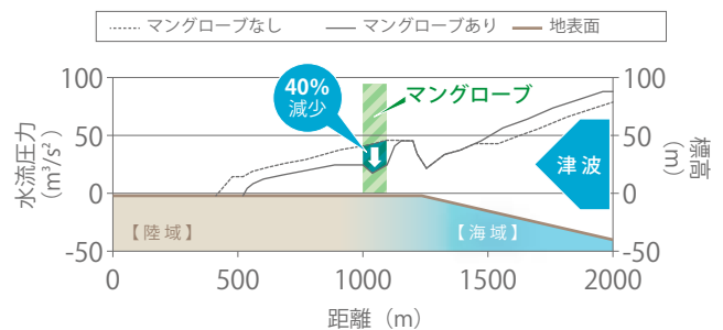
図8 マングローブ林による津波減衰効果(水流圧力) (出典：柳澤ほか, 2010)
