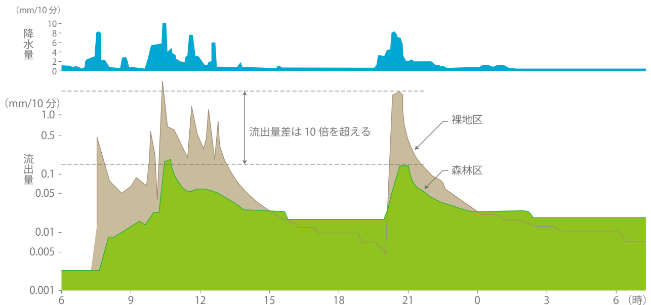
図6 森林と裸地の洪水時流出量の比較事例（出典：福島，1977）
