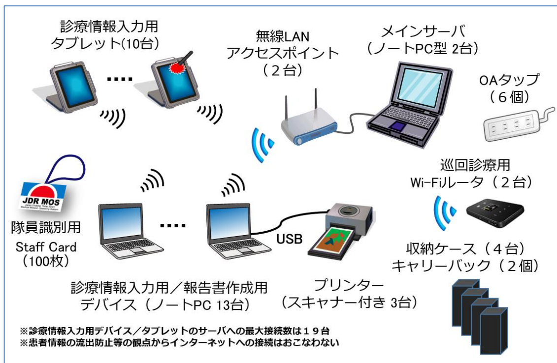
図表：現行 MOS のシステム構成
