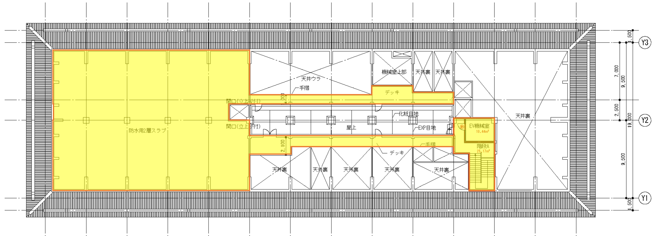
中3階平面図
