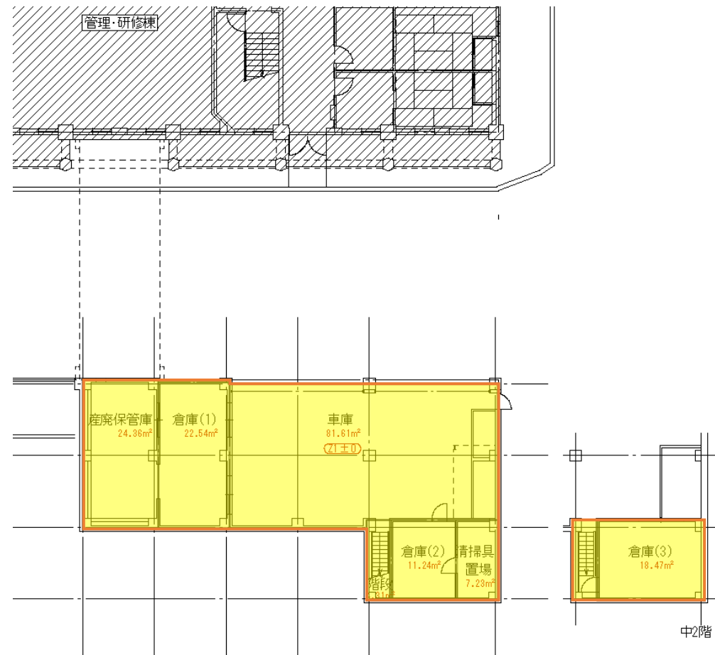
1 階平面図
