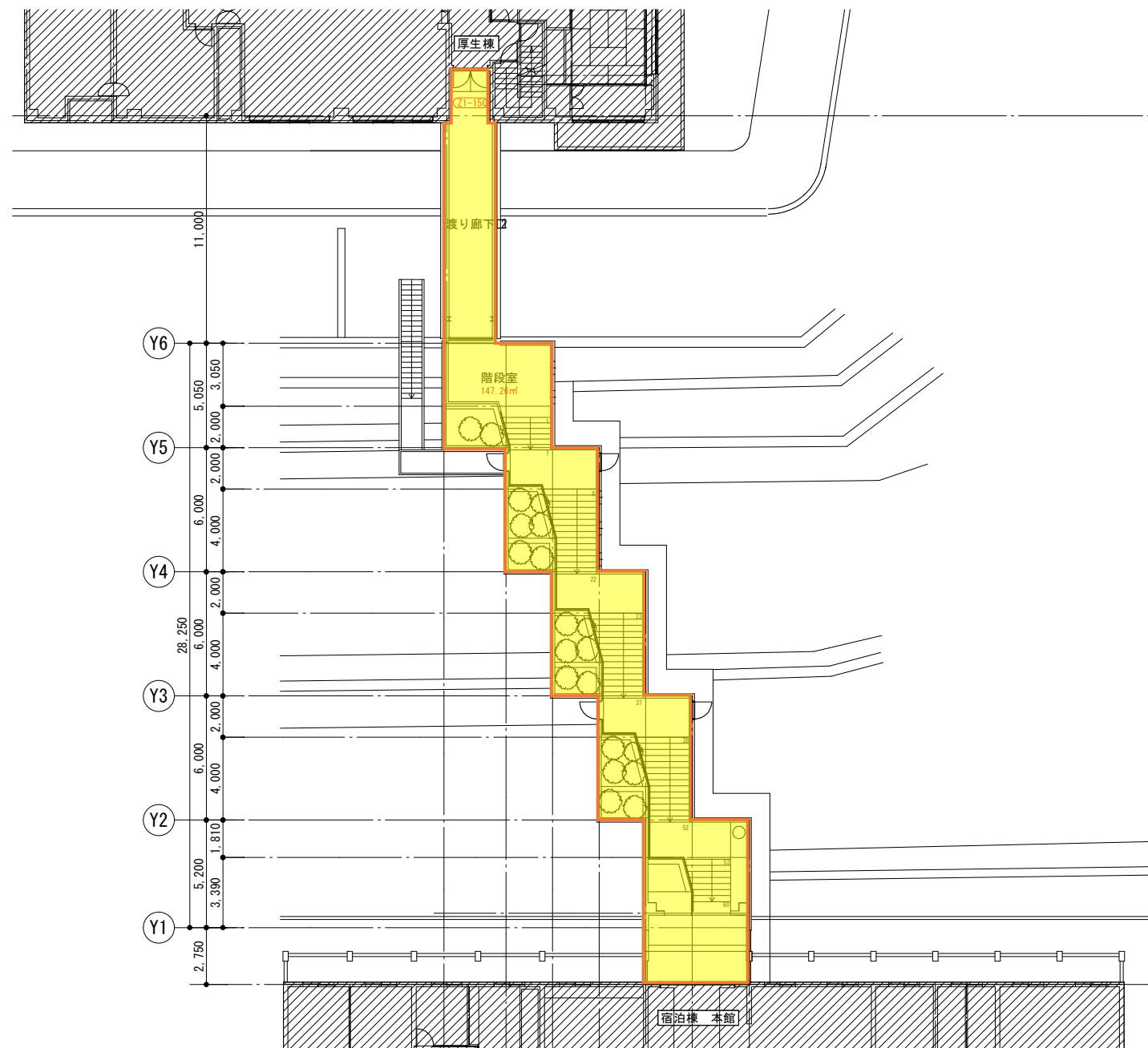
平面図
