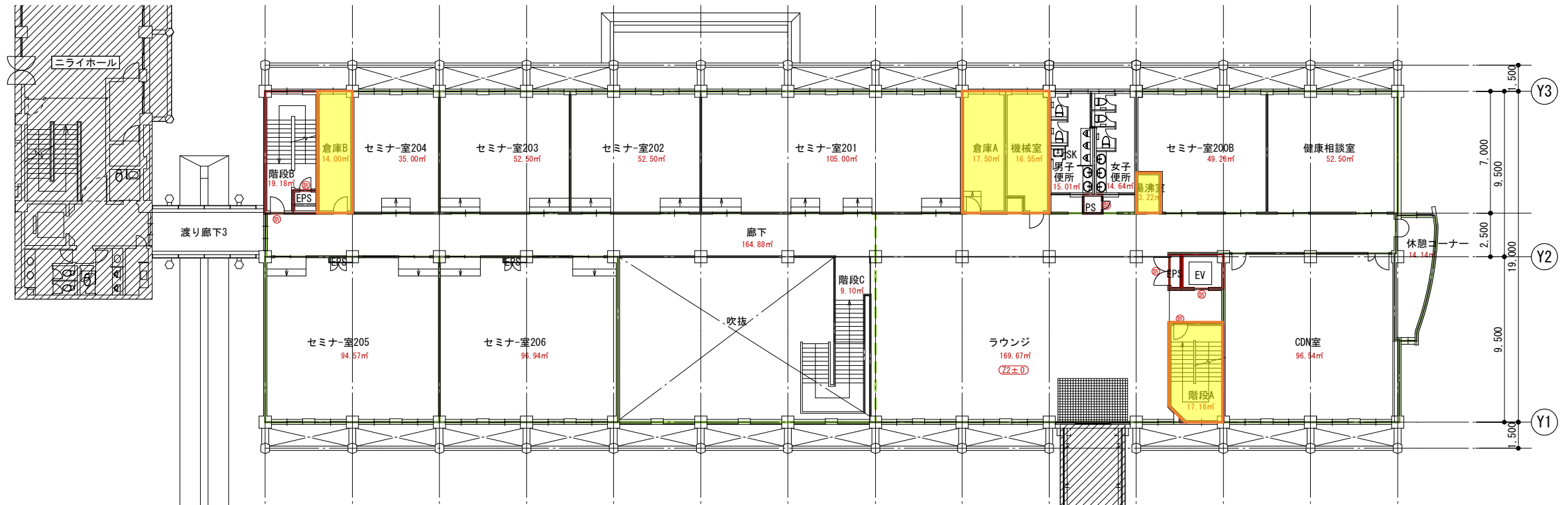
2 階平面図
