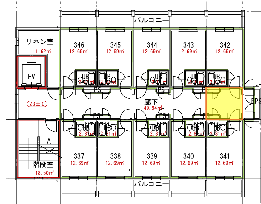
3 階平面図
