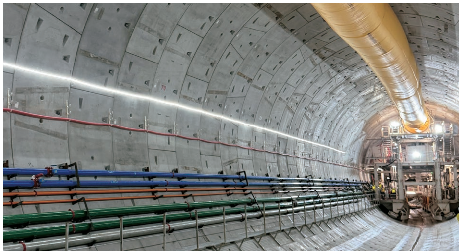
パナマで建設が進む地下鉄のシールドトンネル掘削現場
