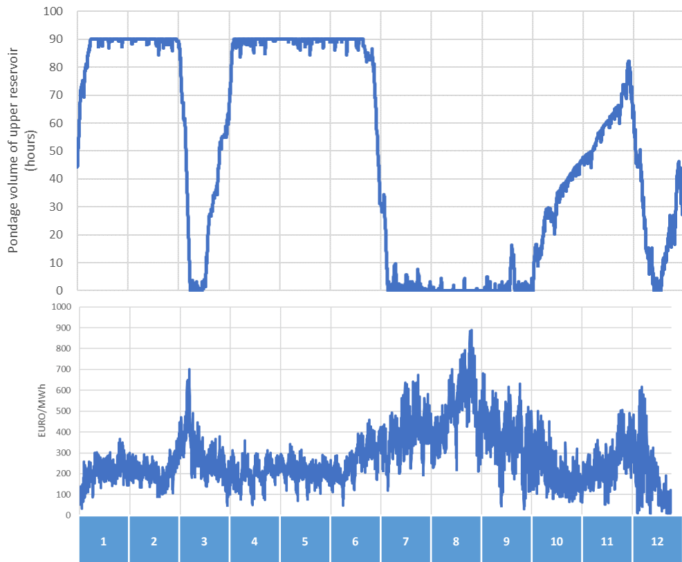
2022年の上部調整池運用模擬結果（上段）と市場価格（下段）
