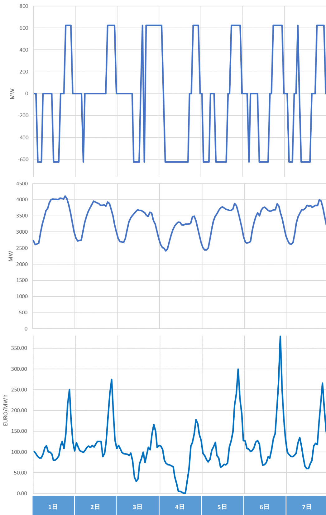
Bistrica揚水発電所の運用模擬結果（上段）、負荷曲線（中段）および市場価格（下段） （2024年8月1日（木）から7日（水））
