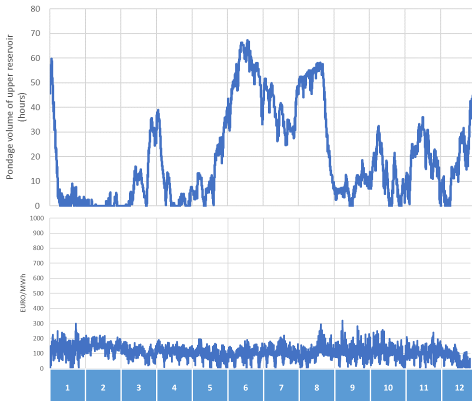
2023年の上部調整池運用模擬結果（上段）と市場価格（下段）
