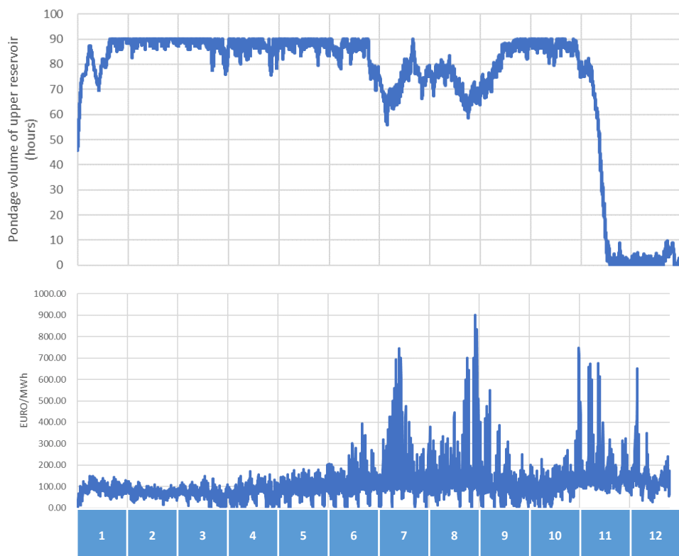
2024年の上部調整池運用模擬結果（上段）と市場価格（下段）
