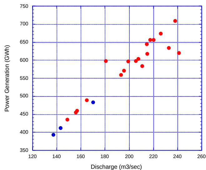
図 3-3 発電設備からの放出水量と発電量
