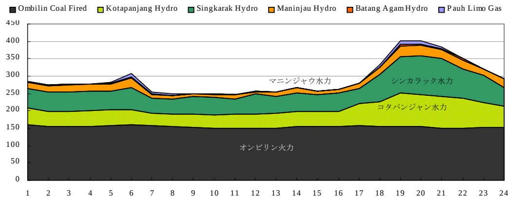
図 3-1 スンバー・リアウシステムの典型的日次負荷曲線 (出典: PLN)
