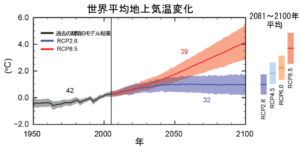
図 9 1986-2005 年平均に対する世界平均地上気温の変化
