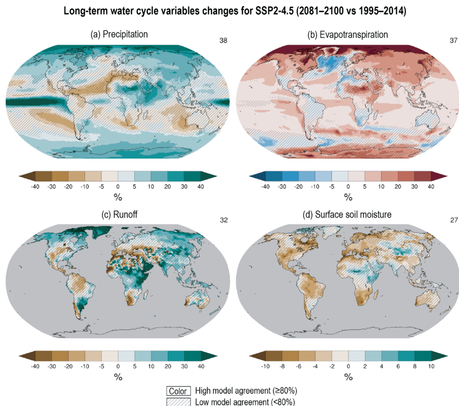
図 11 予測される水循環の変化 20
