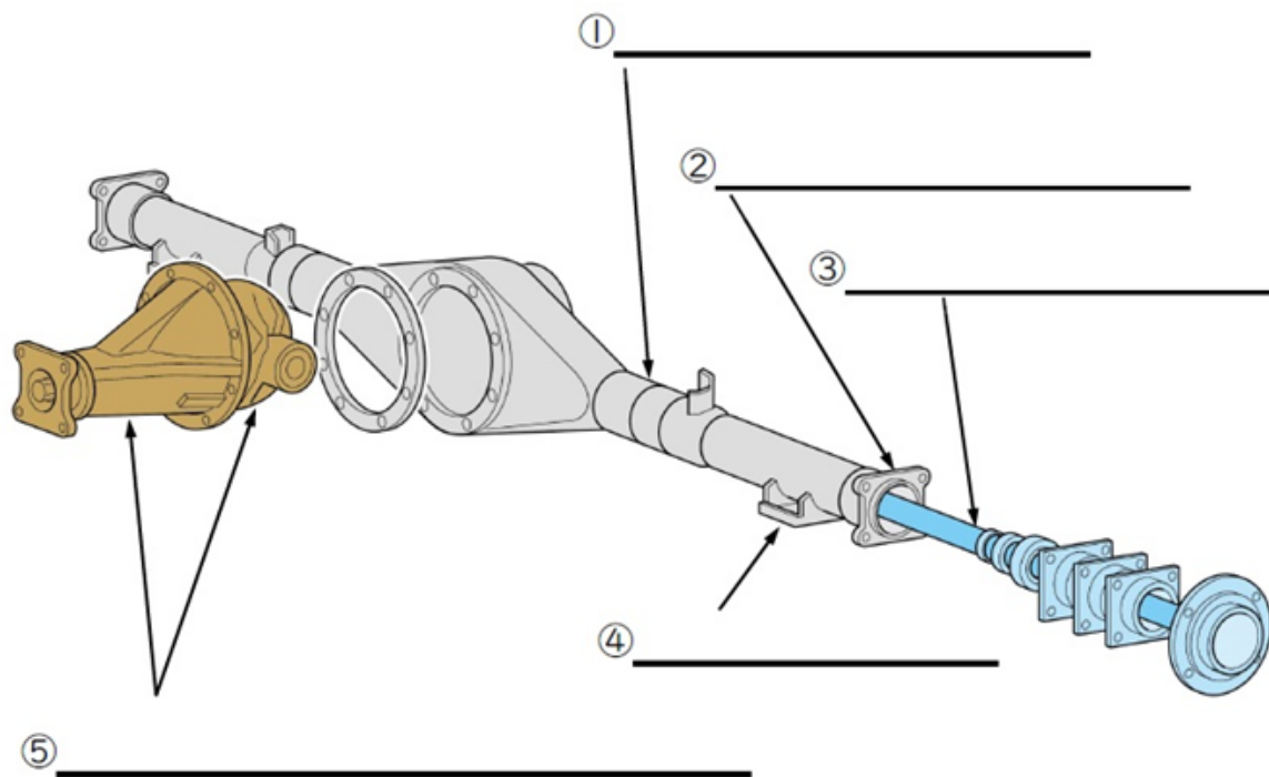
ず しゃじくけんかしき りあ・あくすは 図 2 6 車軸懸架式のリア・アクスル
