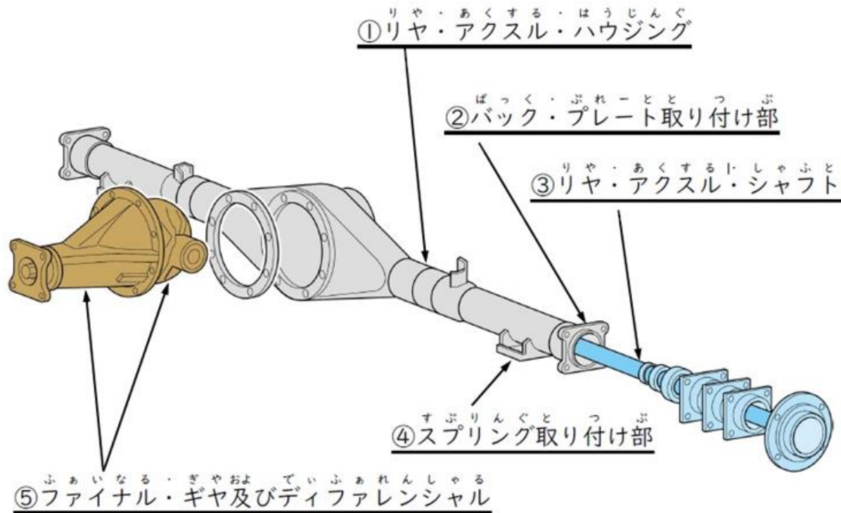
図26 車軸懸架式のリア・あくする
