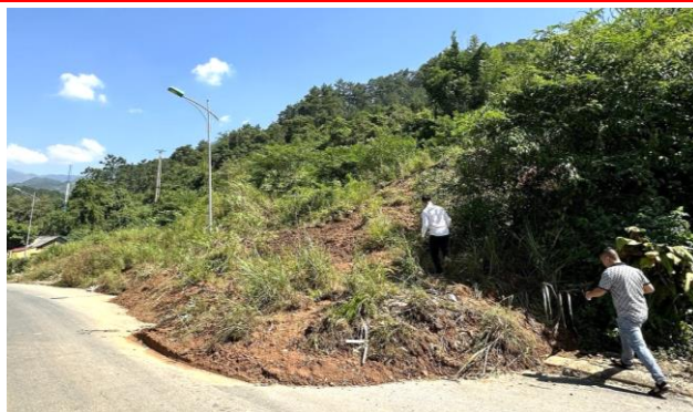
【民間連携事業】地すべり移動土塊が道路へ到達 （奥山ボーリング株式会社）
