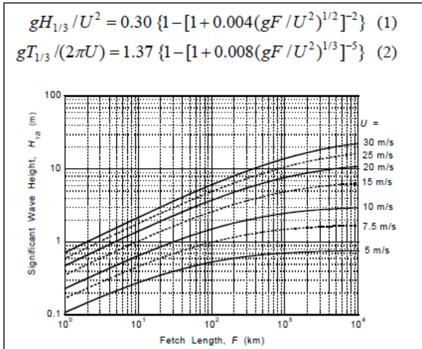
Gráfico 4.17 Relación entre altura representativa de ola y distancia sobre la cual sopla el viento
