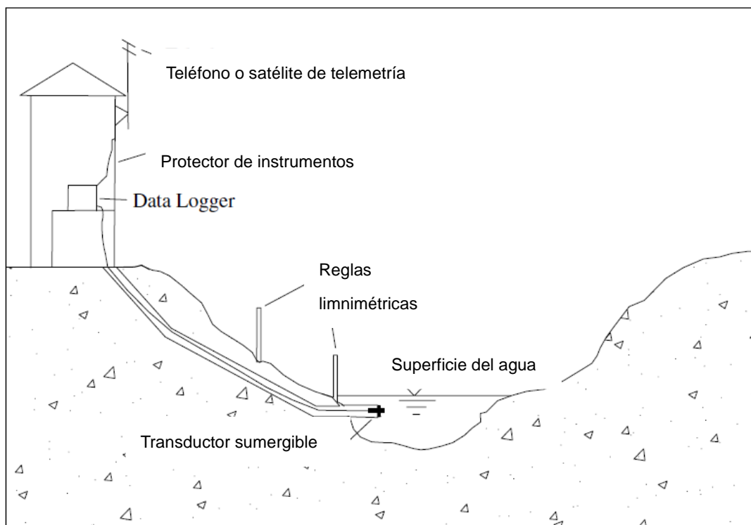
Gráfico 4.21 Esquema de diseño de la instalación del medidor de nivel de agua (Referencia 4.3)
