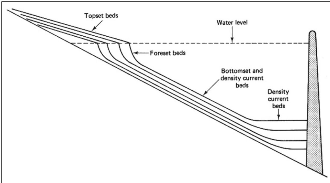
Gráfico 3.7 Patrón Longitudinal de Sedimentación en la Operación de Reservorio con Nivel de Agua Constante (SDSU)
