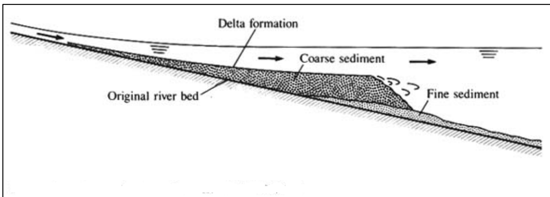
Gráfico 3.6 Deposición de Sedimentos en un Reservorio
