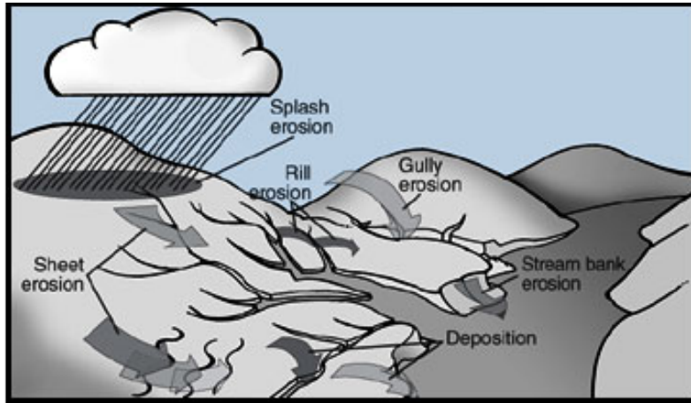
Gráfico 3.1 Tipos de erosión (Referencia 3.1)
