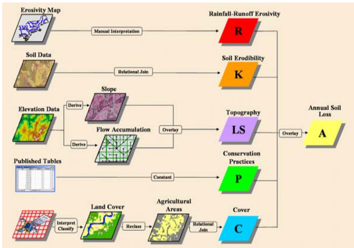
Gráfico 3.3 Cálculo de la Pérdida Anual de Suelo por RUSLE (Universidad de Vermont)
