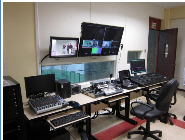
Equipos de TDT que se instalarán en el INICTEL
