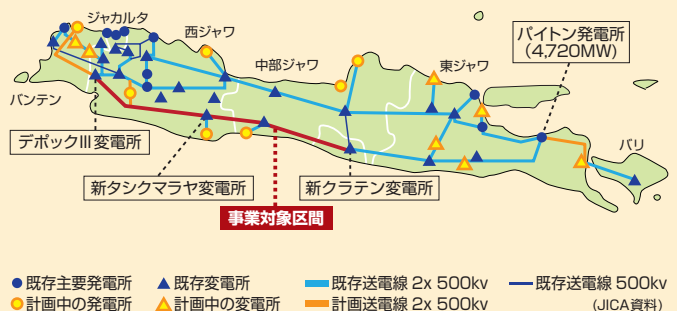
2: ジャワ・バリ系統(デボック・タンクマラヤ間)500kV送電線 (Photo: PT.Perusahaan Listrik Negara)
